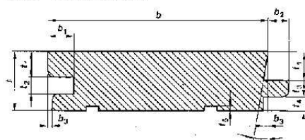
FIG. 1 - Elemento tipo 1
