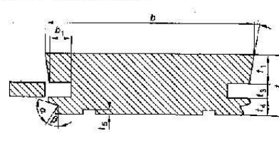
FIG. 2 - Elemento tipo 2
